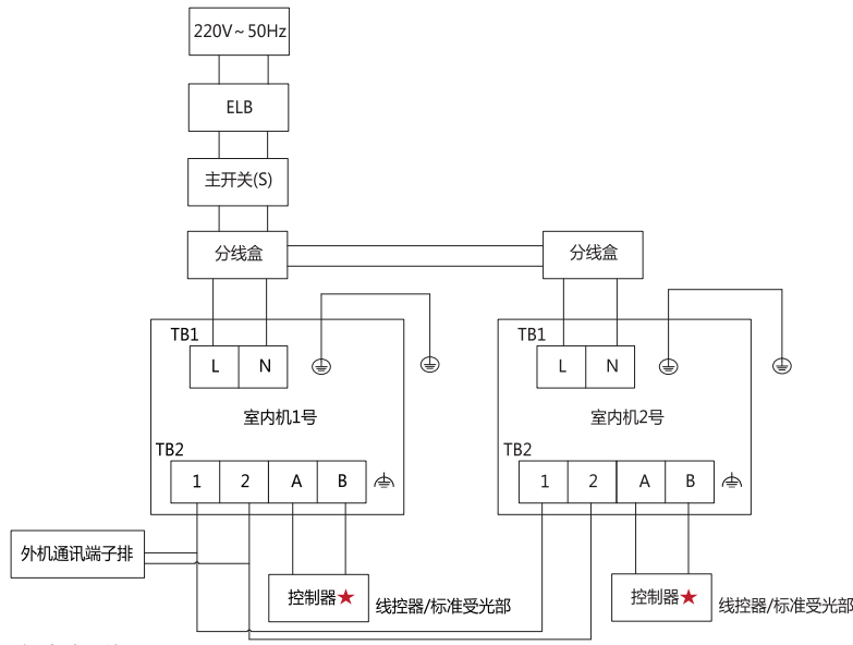
图4 室内机电线的连接
