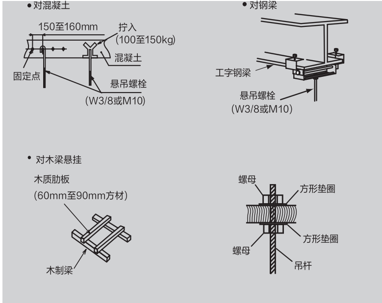
图3 悬吊螺栓的固定
