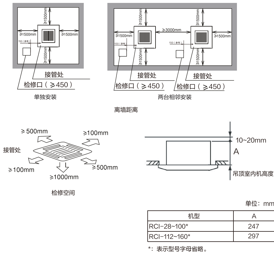
图1 操作和维护空间
