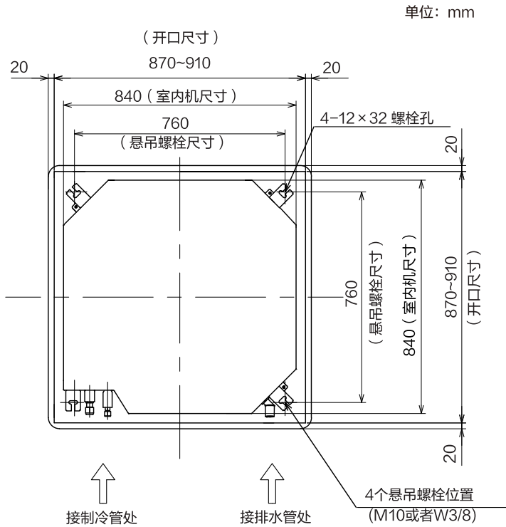
图2 天花板开口及悬吊螺栓位置
